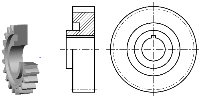
26.3. ábra. Hengeres fogaskerék térhatású ábrája, és műszaki rajza
