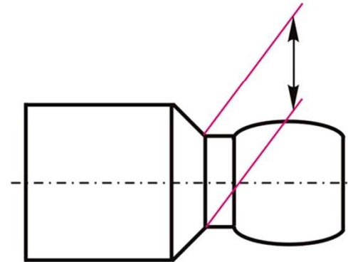
Átlósan kiemelt méretvonalak
